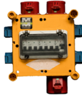
400v Verdeler 32 Ampère
